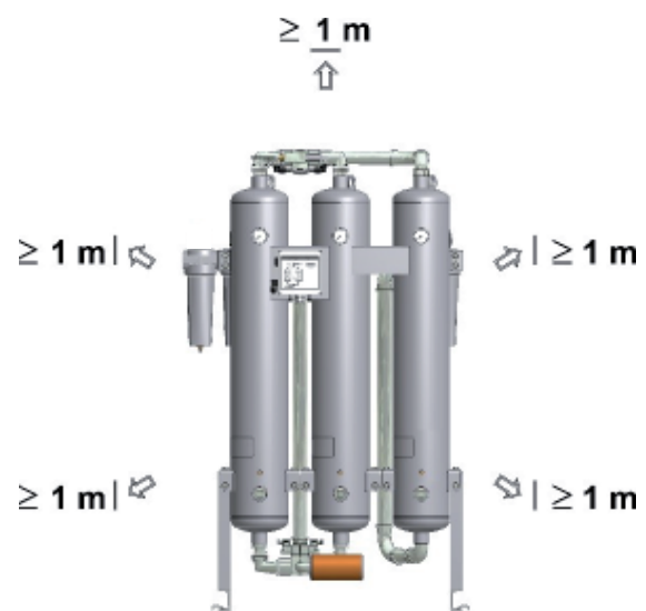
Distancia requerida hacia arriba y a los lados = mín. 1 m
