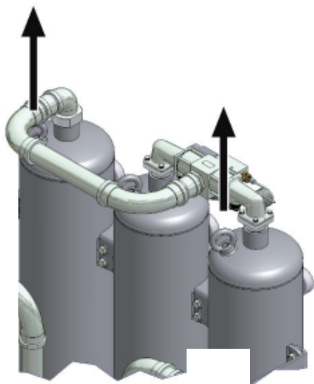
I: Ojo de suspensión en el depósito a presión
